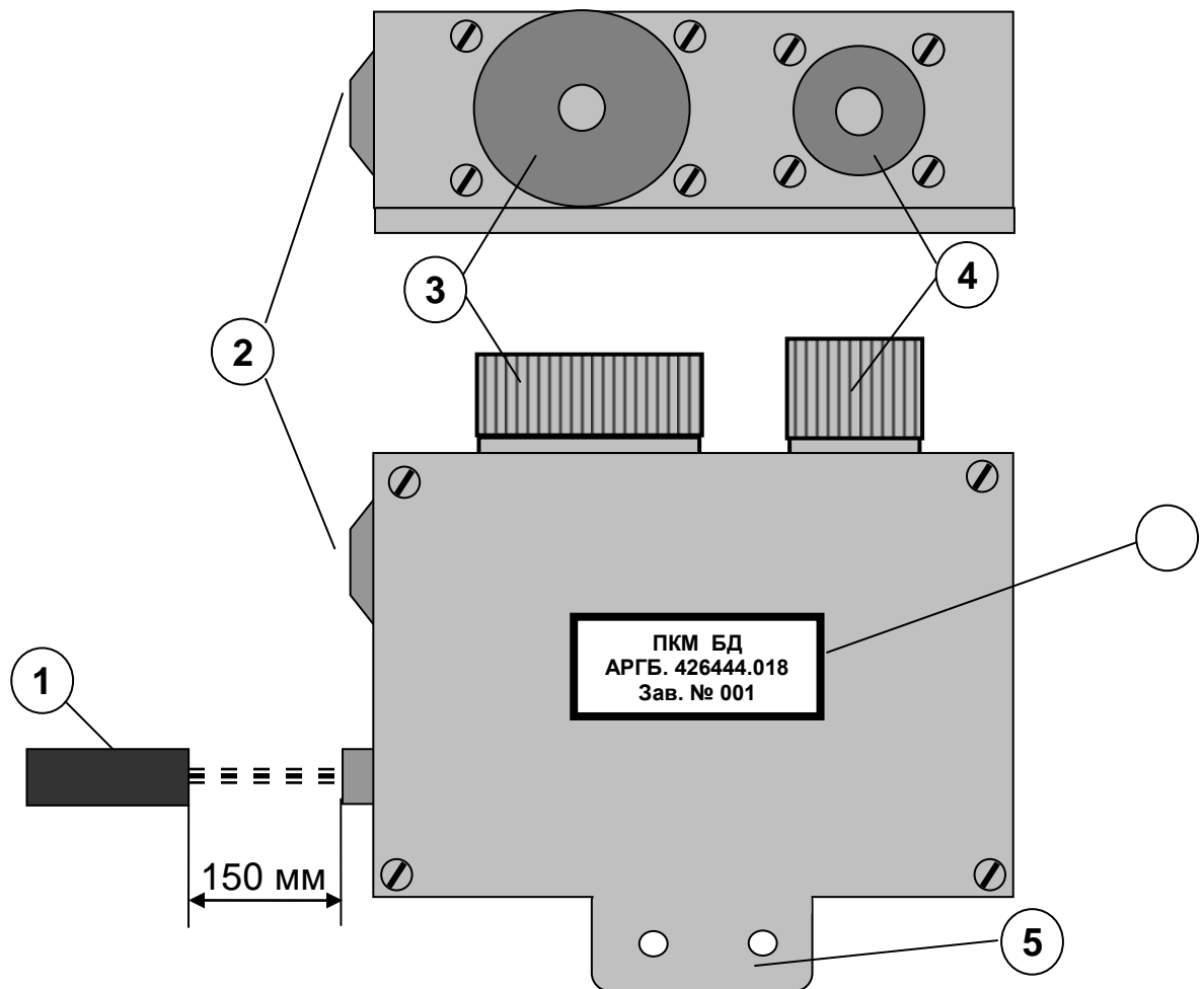
Рисунок 2. Элементы конструкции БД.
